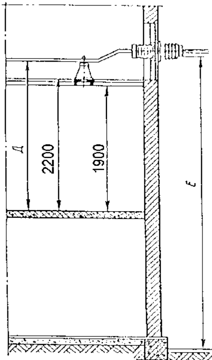
Фиг. 21. Минимални разстояния от неограничени тоководещи части и от долния ръб на изолаторите до пода; светла височина на коридора в ЗРУ; минимални разстояния от неограничени линейни изводи от ЗРУ до терена във външната територия на ЗРУ при липса на достъп на превозни средства под изводите
